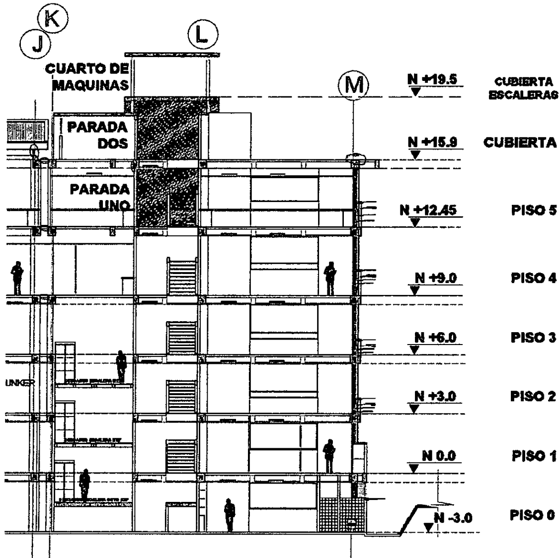
CORTE C-C
