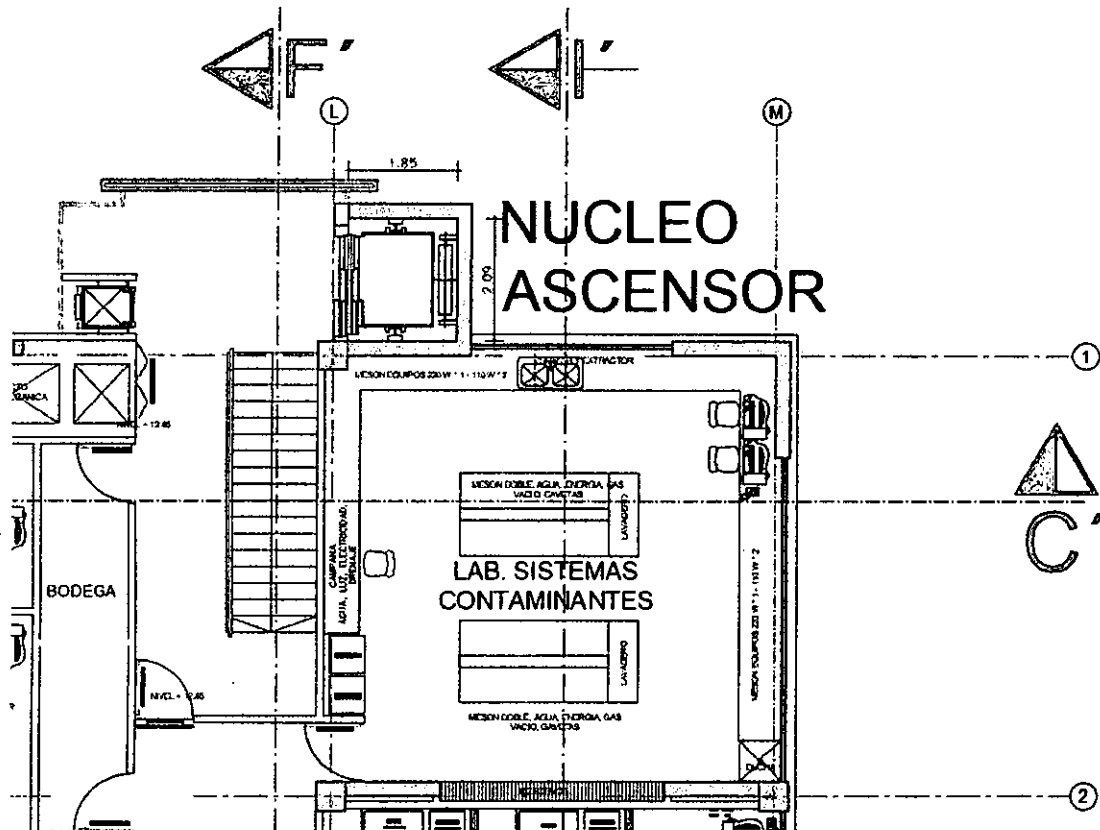
DETALLE PLANTA NÚCLEO ASCENSOR
