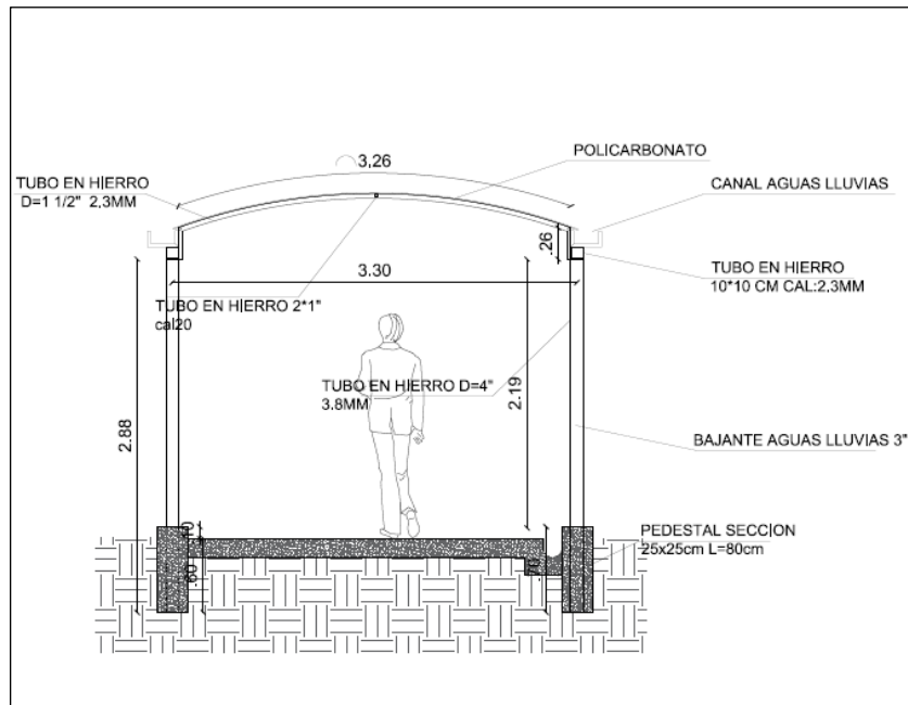
PLANO 2 – DETALLE DOMO FRENTE BLOQUE ADMINISTRATIVO
