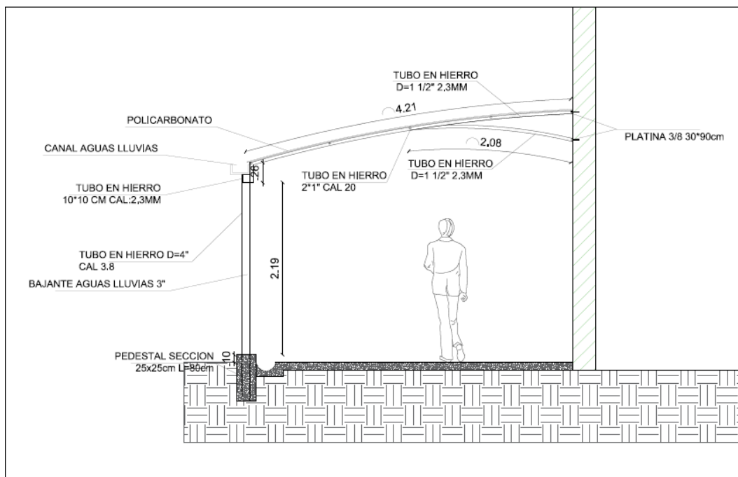
PLANO 3 – DETALLE DOMO BLOQUE DERECHO
