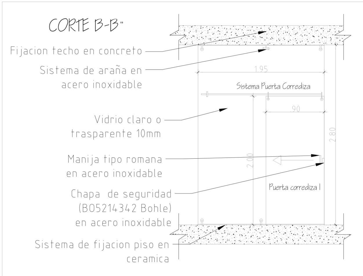
Plano 4 - División tipo 2
