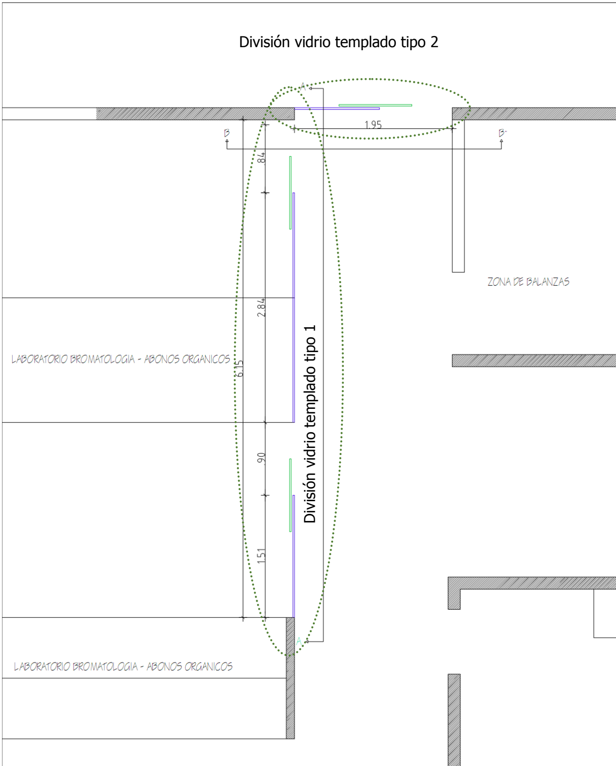
Plano 2 - Detalle Divisiones tipo 1y 2
