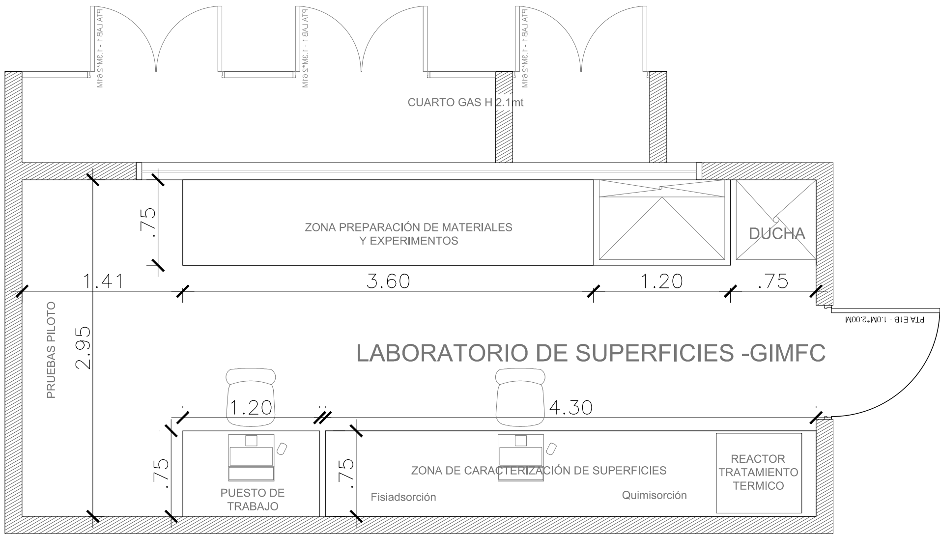
PLANTA ARQUITETONICA LABORATORIO DE SUPERFICIES -GIMFC LABORATORIOS ESPECIALIZADOS
