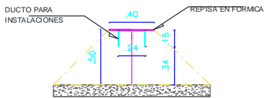
CORTE TRANSVERSAL
