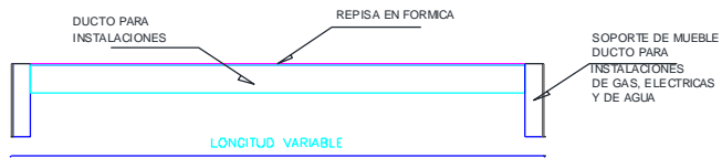
CORTE LONGITUDINAL
