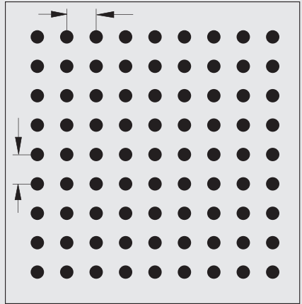
No. 106 ø 2.5 mm. 16% ABIERTO. — 5.50 mm. ↓ 5.50 mm.
