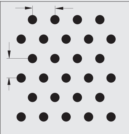
No. 110-M1 ø 3.9 mm. 10% ABIERTO. — 9.43 mm. ↓ 8.15 mm.
