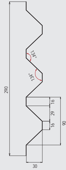
SECCIÓN PANEL MULTILINES 90/30 T
