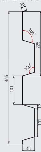
SECCIÓN PANEL MULTILINES 225/45 C
