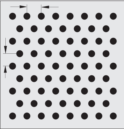
No. 103 ø 2.95 mm. 20% ABIERTO. — 6.30 mm. ↓ 5.45 mm.
